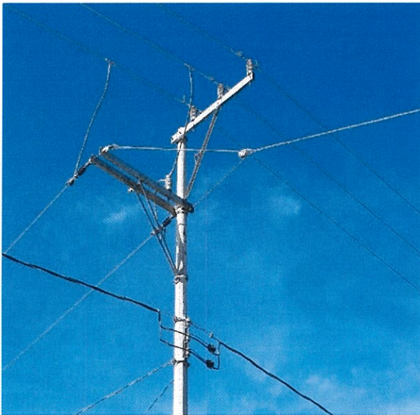
Ampliación de red de Distribución de energía eléctrica, Barrio San Sebastián, La Independencia
